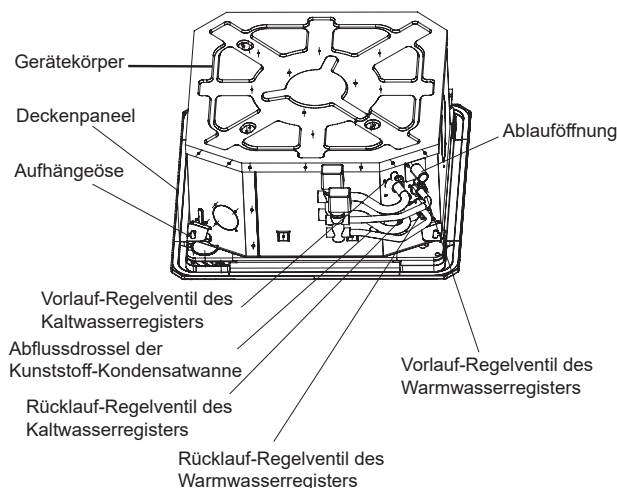
Vierwege-Deckenkassette (kompakt)
